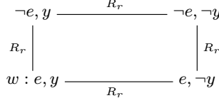
Fig. 2. Spyware example
